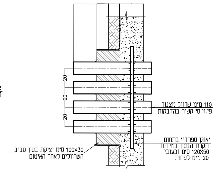
פרט שיוכי מזגן לכויר מזגן מפיץ לכויר
