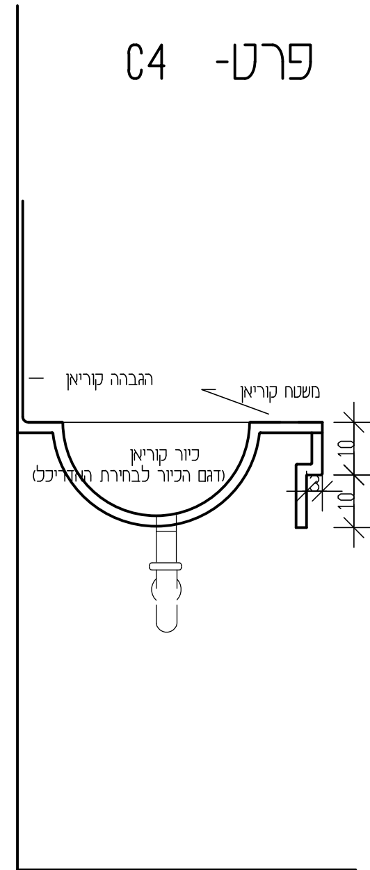
חתיך C4- אנכי במשטח קוריאן עם כיוור עם סינור קידמי מדורג ק.י.מ 1:10
